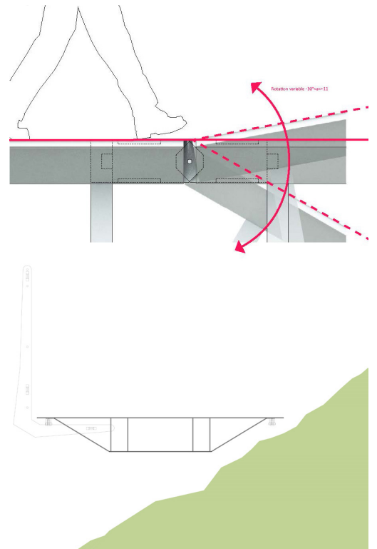
Langsnið sem sýnir öxultengingu og þversnið sem sýnir stígin í hallandi landslagi og festingar fyrir handrið
